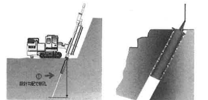
図—5 クローラドリルで削孔
