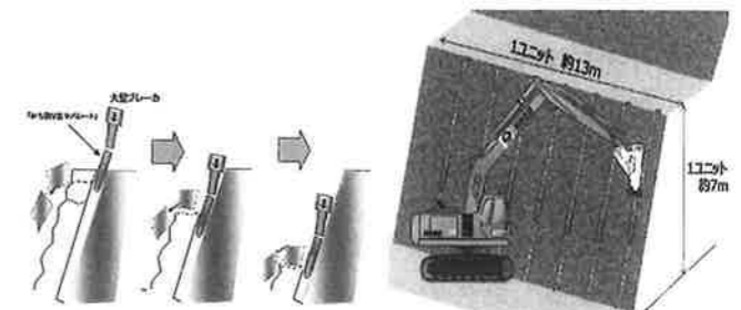
図—3 楔の原理で間接打撃破碎
