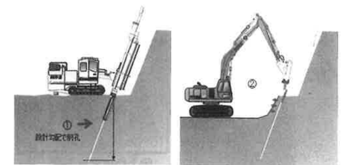
図—1 クローラドリルで削孔
